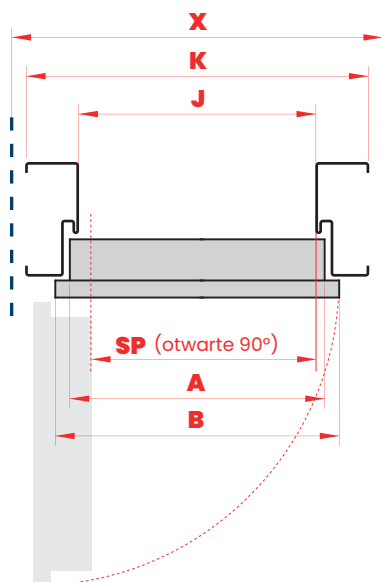
PRZĘKÓJ POZIOMY
