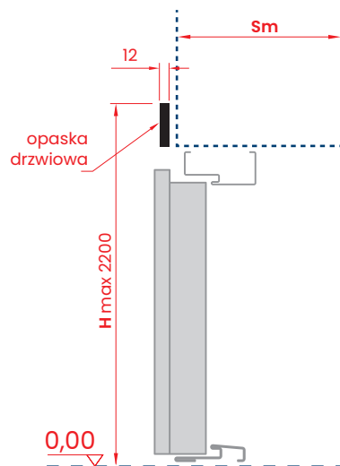
PRZEKRÓJ PIONOWY
