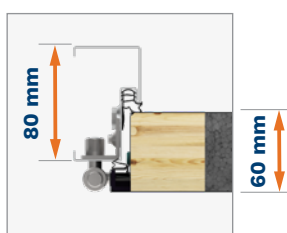
Ościeżnica PERFOTHERM 60
